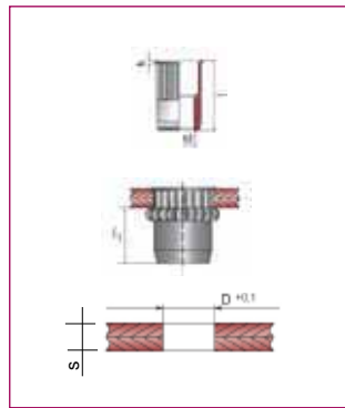
Blindnietmutter Universal-E Edelstahl 1.4570/1.4303 Ecrou en acier universel-S pour rivet aveugle Blind rivet nut Universal-E Grade A2 (304) Rivetti a strappo universali E in acciaio inox Universal-E 304 paslanmaz çelik somun perçin
