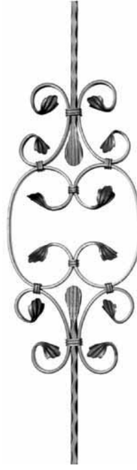
Best.-Nr. 5318 250 x 340 mm 2,45 kg
