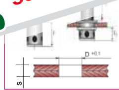
Blindnietgewindebolzen Rifbolt-E Edelstahl 1.4570/1.4303 Boulon en Inox 304 Rifbolt-E pour rivet aveugle Blind rivet bolt Rifbolt-E Inox 304 Vite in acciaio inox 304 Rifbolt-E per ribattini ciechi Rifbolt-E 304 paslanmaz çelik vida perçin
